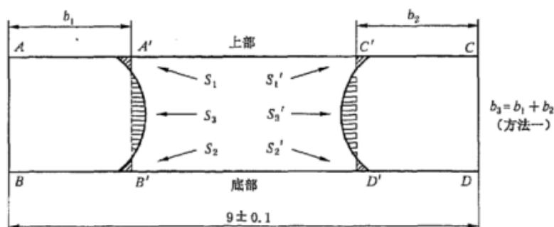
图 4 德尔夫特试样割口剖面图
