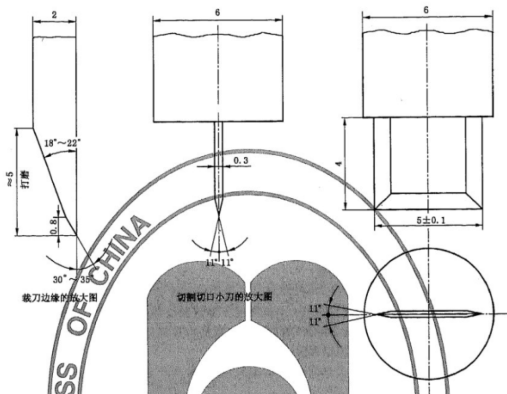
图2 德尔夫特撕裂试样裁刀刃口放大图
